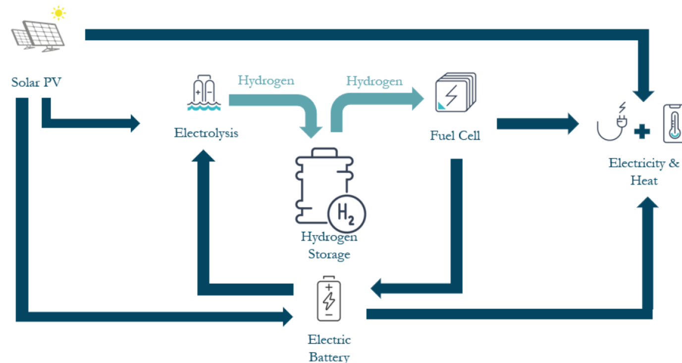
Sistema de reserva de energía a base de hidrógeno
